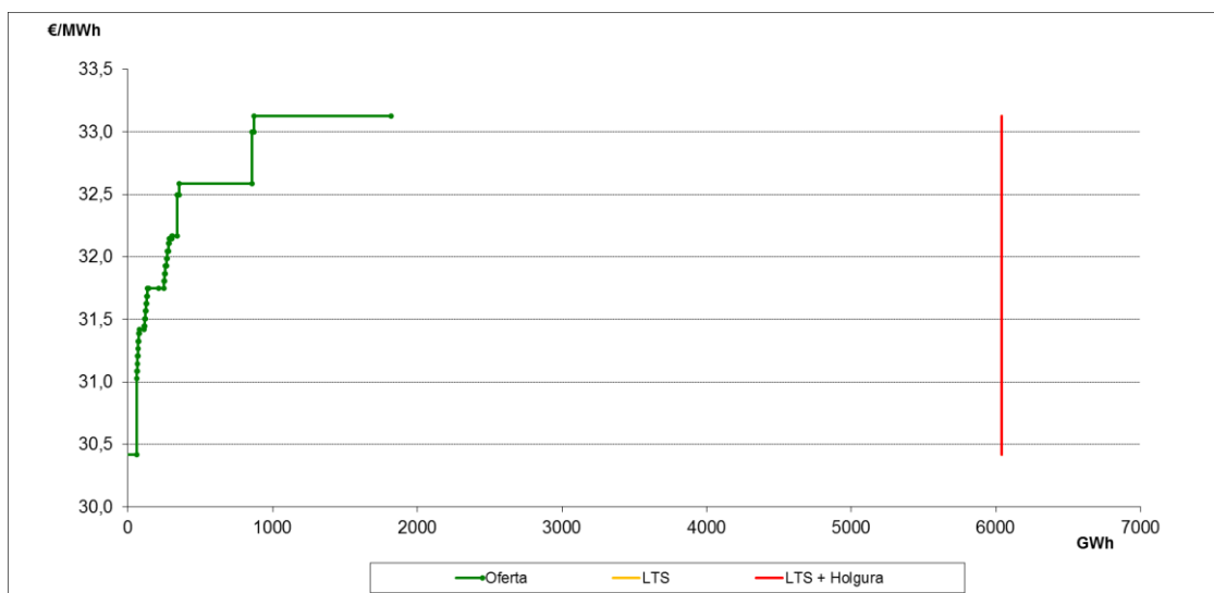
Curva agregada de casación del periodo 2 (16/08/2013 - 31/10/2013)
