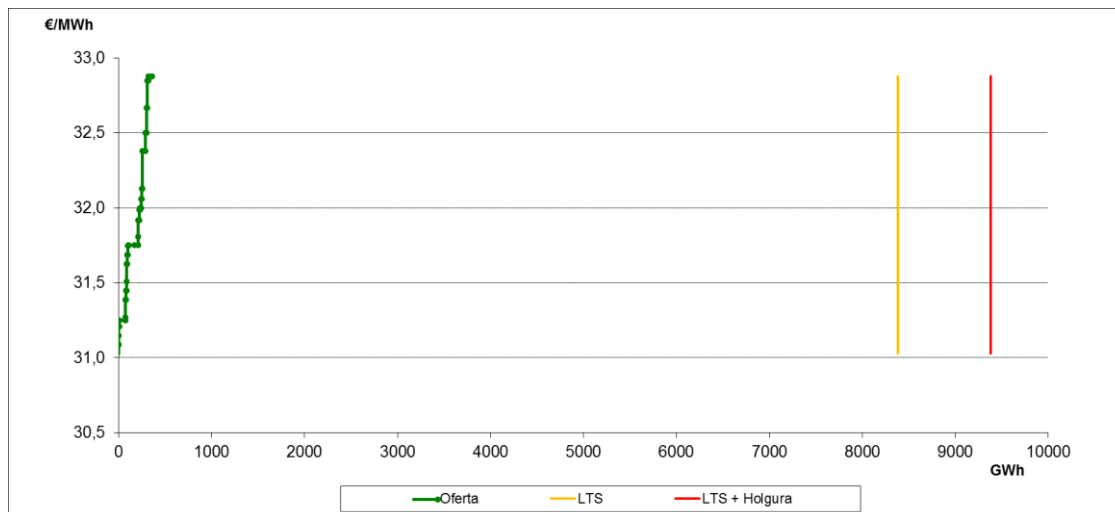
Curva agregada de casación del periodo 1 (01/06/2013 - 15/08/2013)
